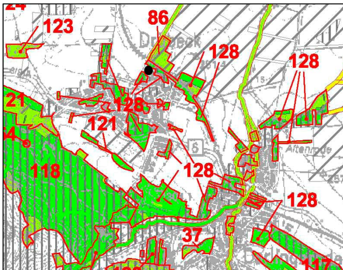
Biotopverbundplanung für die Umgebung des Plangebietes (schwarzer Punkt), Ausschnitt
